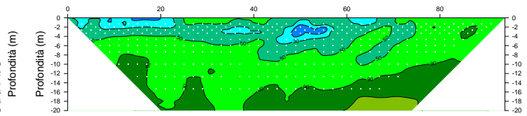
Resistività apparenti misurate - dipoli diretti
