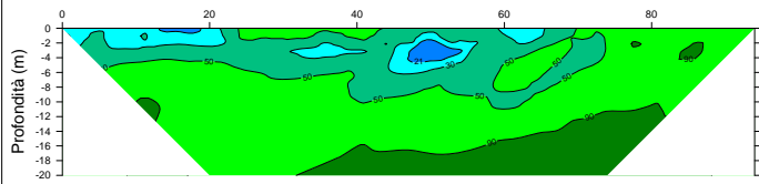
Resistività apparenti calcolate - dipoli diretti
