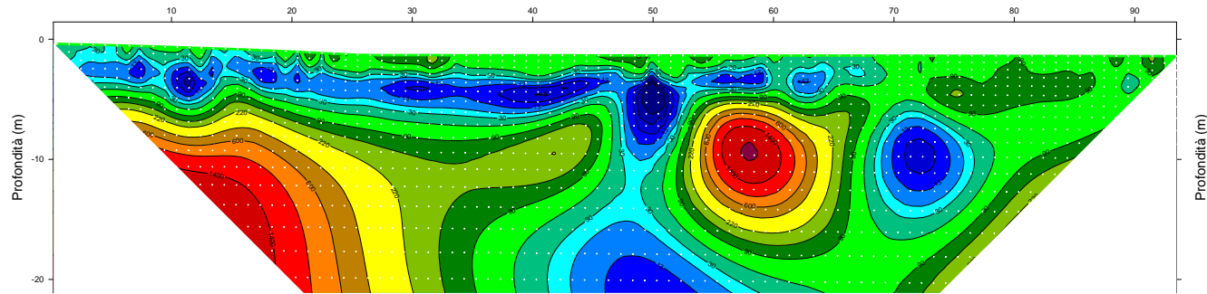
Modello di resistività reali del terreno
