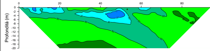
Resistività apparenti calcolate - dipoli inversi
