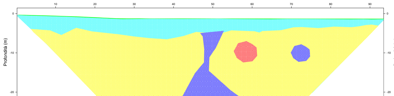
Interpretazione del modello di resistività
