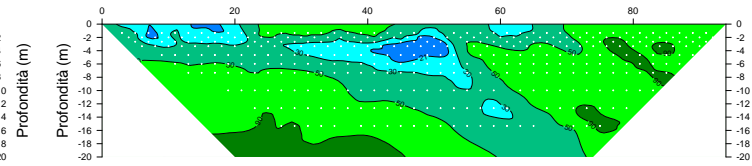
Resistività apparenti misurate - dipoli inversi
